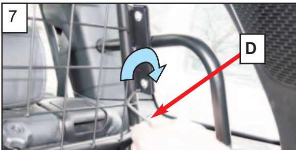
7 Tighten bolts. Repeat for R/H side Schrauben festziehen. Wiederholen Sie dies für die R/H Seite
