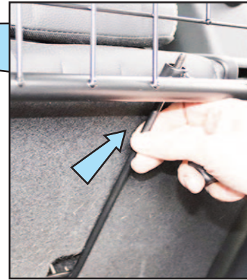
4 Insert bolts 'C'. Schrauben 'C' einsetzen
