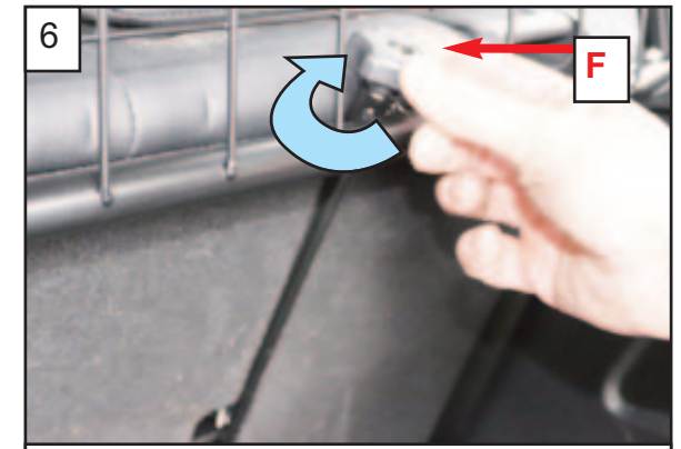
6 Tighten lower fixing hooks. Repeat for L/H side Die unteren Befestigungshaken festziehen. Wiederholen Sie dies für die L / H Seite
