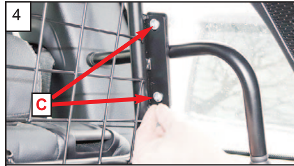
4 Insert bolts 'C'. Schrauben 'C' einsetzen
