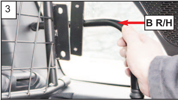
3 Insert R/H side arm. Setzen Sie den R / H-Seitenarm ein.
