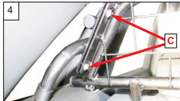
4 Insert bolts 'C'. Do not fully tighten Schrauben 'C' einsetzen.
