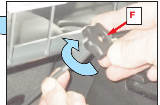
Tighten lower fixing hooks. Repeat for L/H side Die unteren Befestigungshaken festziehen. Wiederholen Sie dies für die L/H Seite
