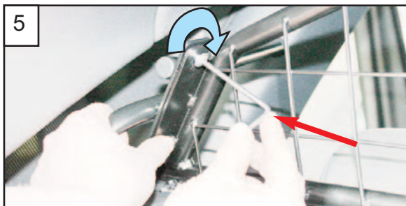
5 Tighten bolts. Repeat for R/H side Schrauben festziehen. Wiederholen Sie dies für die R/H Seite
